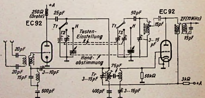
Bild 8. UKW-Eingang mit zwei UKW-Tasten plus UKW-Handabstimmung (Blaupunkt-Paris)
