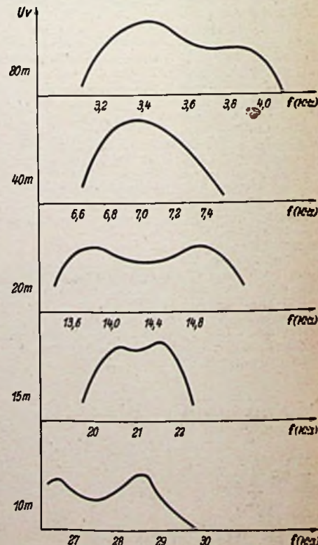
Bild 4. Spannungskurven eines Bandfilter-Steuersenders
