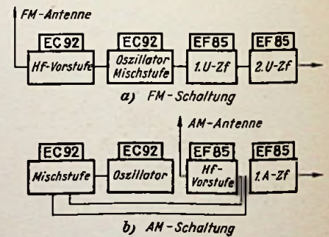
Bild 4. Röhrenausschaltung im Blaupunkt Paris
