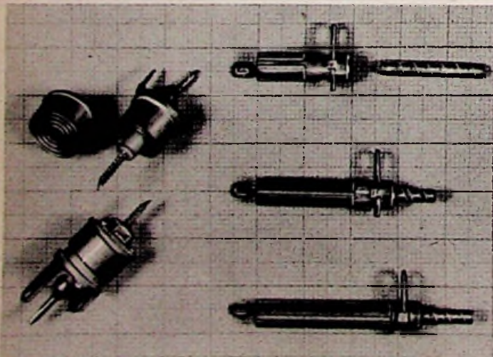
Bild 3. Philips-Lufttrimmer (30 pF) und keramische Rohrtrimmer (5, 10, 18 pF)
