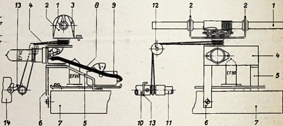
Anordnung der Ferritstab-Antenne bei einem Grundig-Gerät
