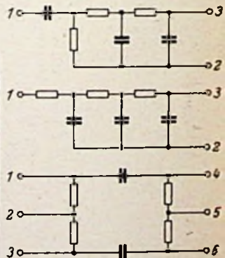
Bild 4. Beispiele von kombinierten Schaltelementen, wie Integrationsglieder in Fernsehempfängern und Diodenfilter für Ratiodetektoren
