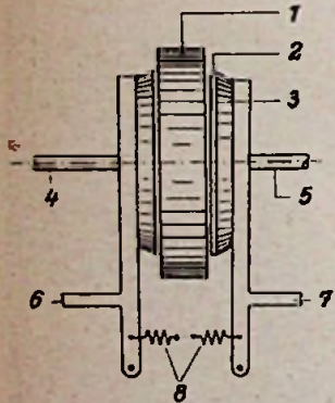
Bild 1. Prinzip der Kupplungs-waage von Siemens. 1 = Schwungmasse, 2 = Kupplungsbelag, 3 = Kupplungs-scheibe, 4 = Antriebsachse für KML, 5 = UKW-Antriebsachse, 6 = zu den Tasten KML, 7 = zur UKW-Taste
