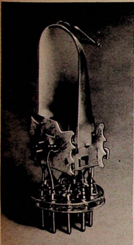
Bild 3. Mechanischer Aufbau des Röhrensystms
