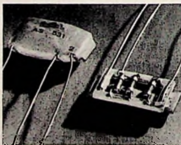
Bild 3. Baueinheiten mit mehreren kombinierten Schaltelementen, um Verdrahtungsarbeit in Empfängern zu ersparen
