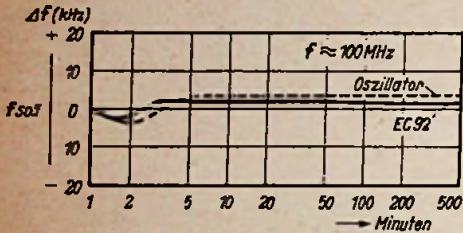
Bild 7. Frequenzverlauf bei einer richtig durchgeführten Kompensation
