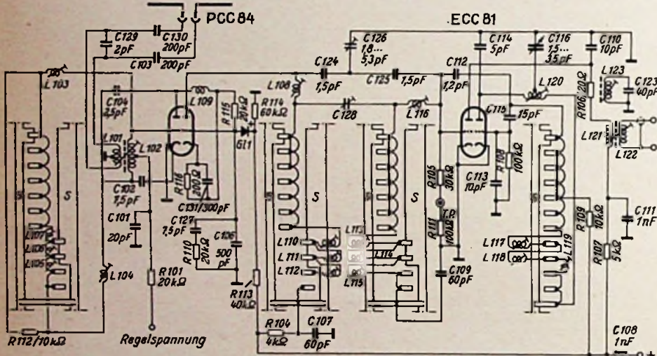
Bild 2. 10-Kanal-Schalter mit Eingangsschaltung von Graetz. Die Schalterkontakte sind als Rechtecke dargestellt. Kontakte und Schaltsegmente S sind geradlinig abgewickelt gezeichnet
