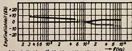
Bild 4. Toleranzwerte für die Frequenzkurve des Dual-Duplo-systems CSD 1
