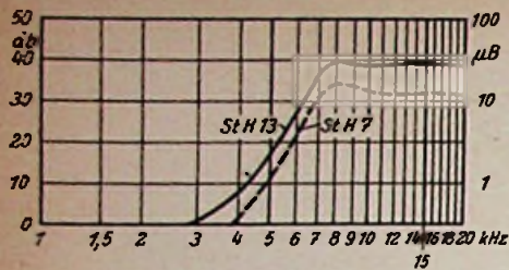
Bild 7. Schalldruckkurve bei LC-Ankopplung, Mikrofonabstand 1 m
