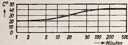
Bild 1. Temperaturänderung am UKW-Oszillator während des Betriebs. Die erste Minute ist als Geräteanlaufzeit weggelassen
