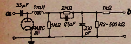
Bild 6. Verbesserter Gegenkopplungskanal
