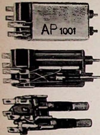
Bild 1. Philips-Mikro-Bandfilter. Oben: AM-Bandfilter AP 1001 im Gehäuse; Mitte: ohne Gehäuse; Unten: FM-Mikro-Bandfilter ohne Gehäuse. Hohe Güte sowie Temperaturfestigkeit bis +90°C sind weitere Kennzeichen dieser Kleinbau-Teile
