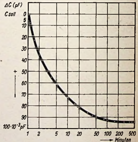
Bild 5. \Delta C -Kurvenverlauf des gesamten Oszillators
