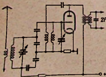
Bild 8. Selbstschwingende Triodenmischschaltung
