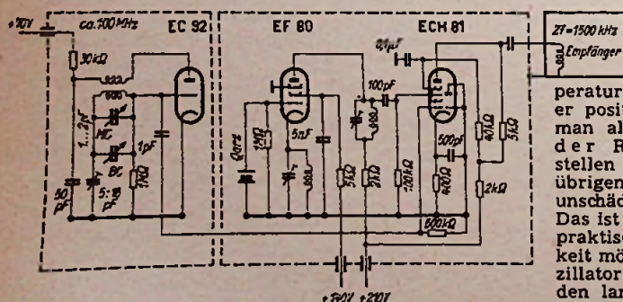
Bild 4. Schaltung der Meßanordnung
