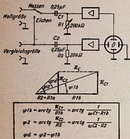
Phasenwinkelmessung mittels zweier RC-Glieder
