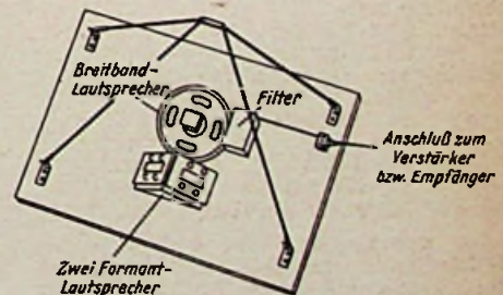
Bild 4. Anordnung der Lautsprecher auf der Schulfunk-Schallwand von Körting mit zwei Formant-Lautsprecher
