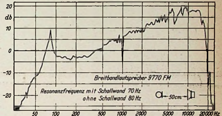
Bild 2. Schalldruckkurve des Breitbandlautsprechers 9770 FM
