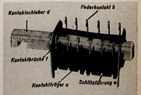
Bild 5. Neuartiger Schiebeschalter (Blaupunkt)
