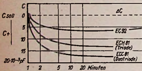
Bild 3. Kapazitäts-Änderung verschiedener Röhren während der Einlaufzeit
