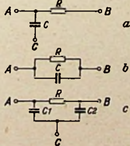
Bild 2. Schaltungen von Gitterkombinationen der NSF
