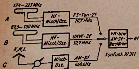
Bild 8. Die drei Eingänge im Tonfunk W 311
