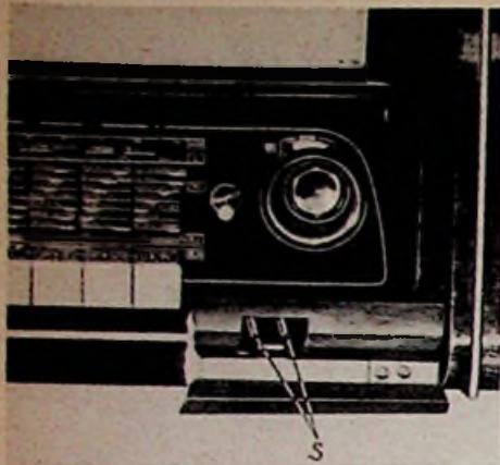
Bild 6. UKW-Stationstasten mit den zugehörigen Einstellschrauben S hinter einer heruntergeklappten Schutzleiste (Blaupunkt)
