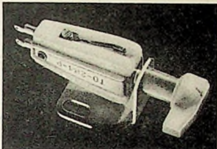
Bild 1. Ronette-Tonabnehmersystem TO 284
