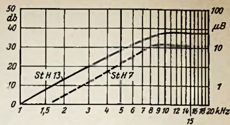
Bild 9. Schalldruckkurve bei RC-Ankopplung, Mikrofonabstand 1 m
