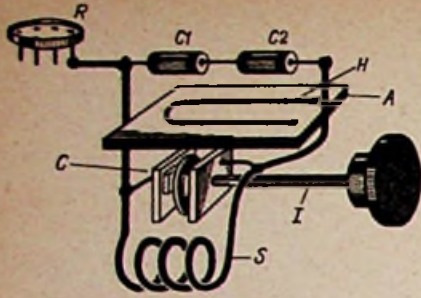
Bild 6. Anordnung der zusätzlich beheizten Kondensatoren mit negativem TK. H = Heizdraht, A = Asbestplatte, C1, C2 = Kondensatoren mit negativem TK, R = Röhrenfassung, C = UKW-Drehkondensator, I = isolierte Achse, S = UKW-Spule
