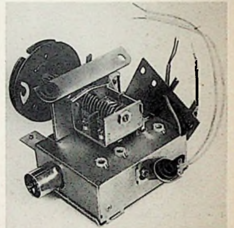
Bild 9. Abgeschirmter Graetz-UKW-Oszillator mit der Röhre EC 92
