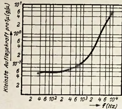
Bild 2. Kleinste Auflagekraft in Abhängigkeit von der Frequenz bezogen auf eine konstante Auslenkung von \mu = 10^{-6} m für das Kristallsystem KST 8 A und C
